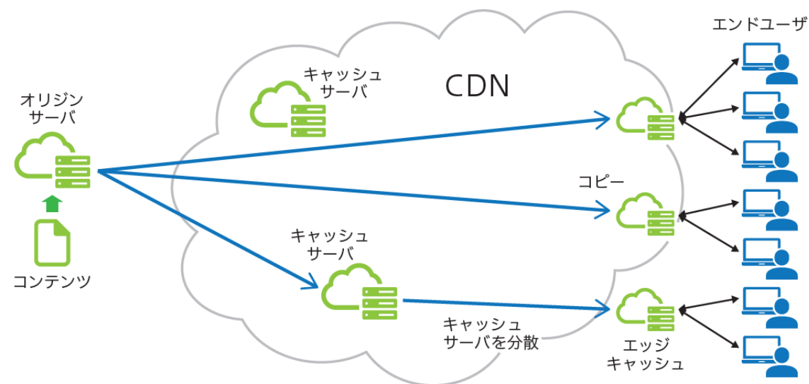
図1 CDNの構成
